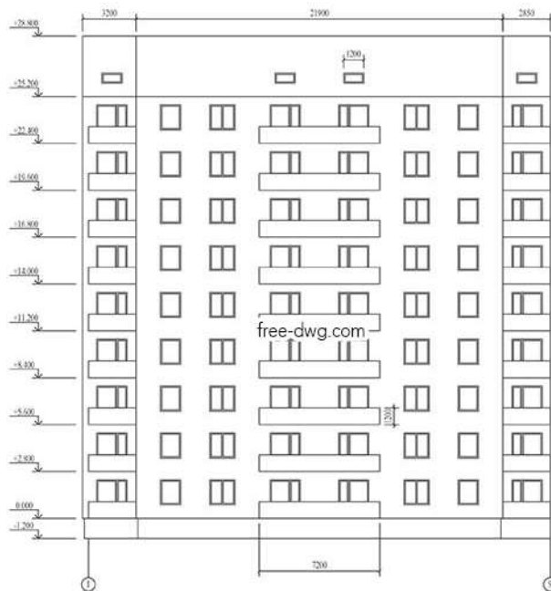
Фасад в осях 1-9
