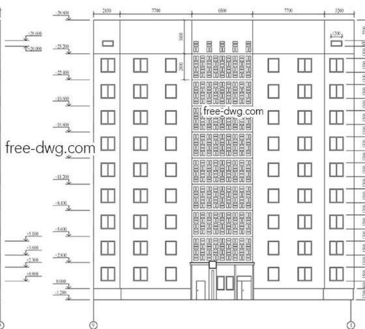
Фасад в осях 9-1
